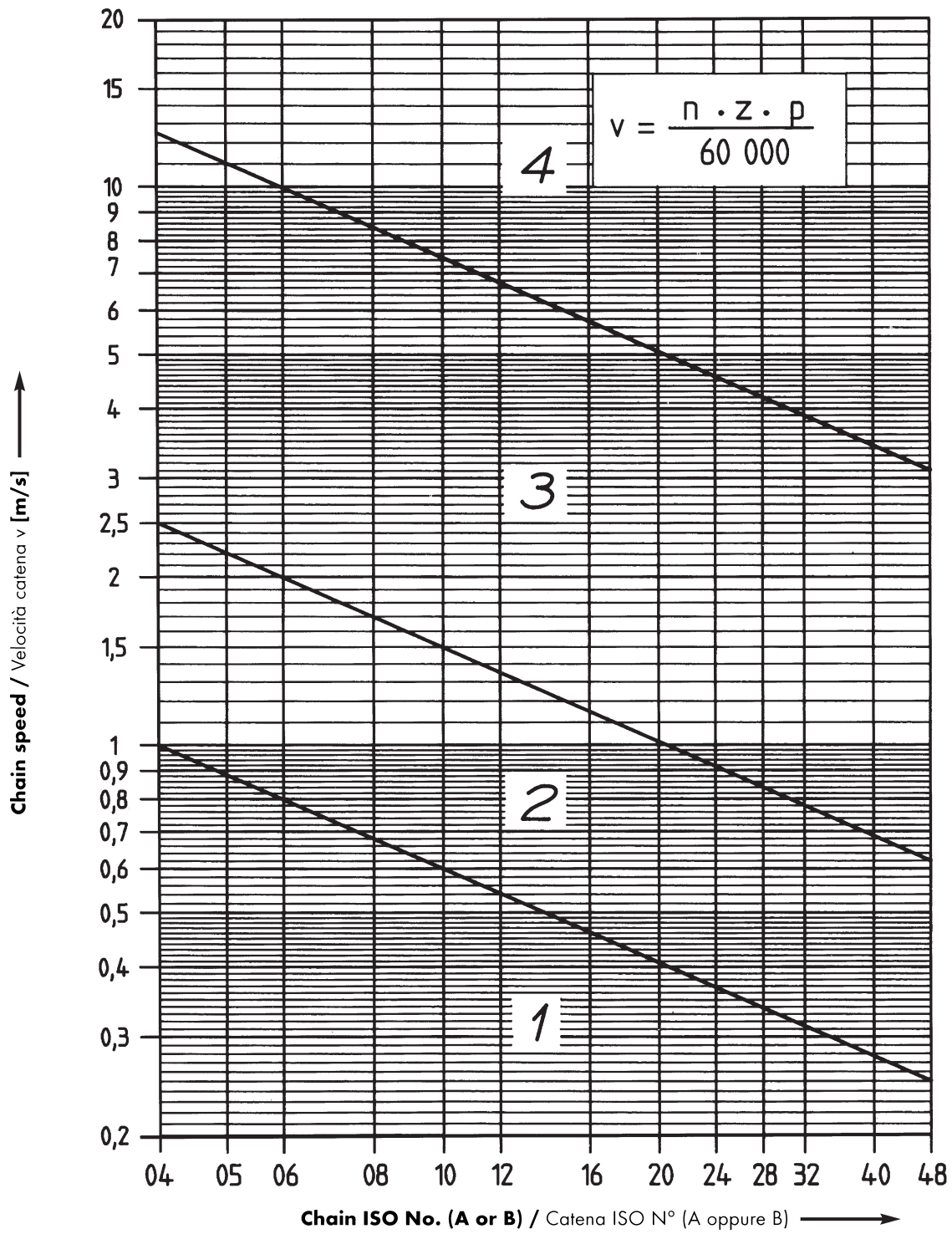
Pict. 4 - Lubrication fields Fig. 4 - Campi di lubrificazione
